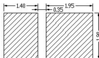
建议焊盘
